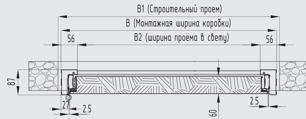
ДВЕРНАЯ КОРОБКА ДЛЯ ВРЕЗНОГО МОНТАЖА
